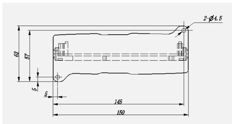
图 1.1 安装底板尺寸图
