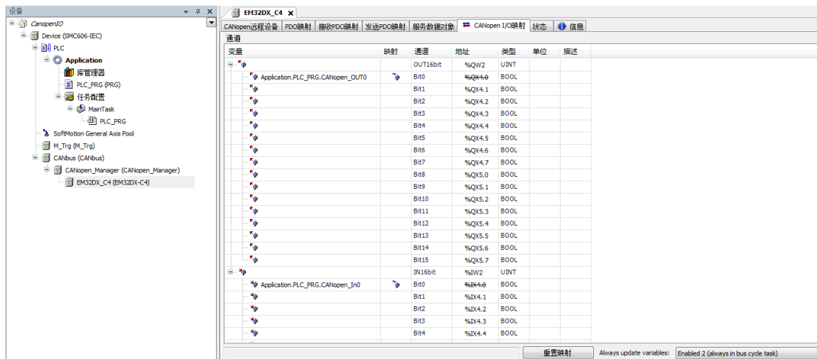
图 5.13 配置 IO 映射页面
