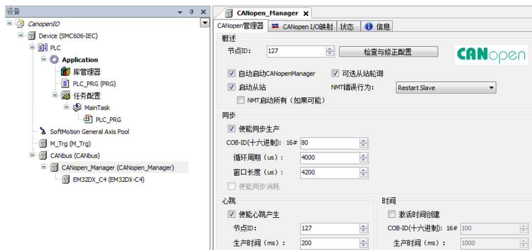
图 5.9 CANopen 主站配置页面
