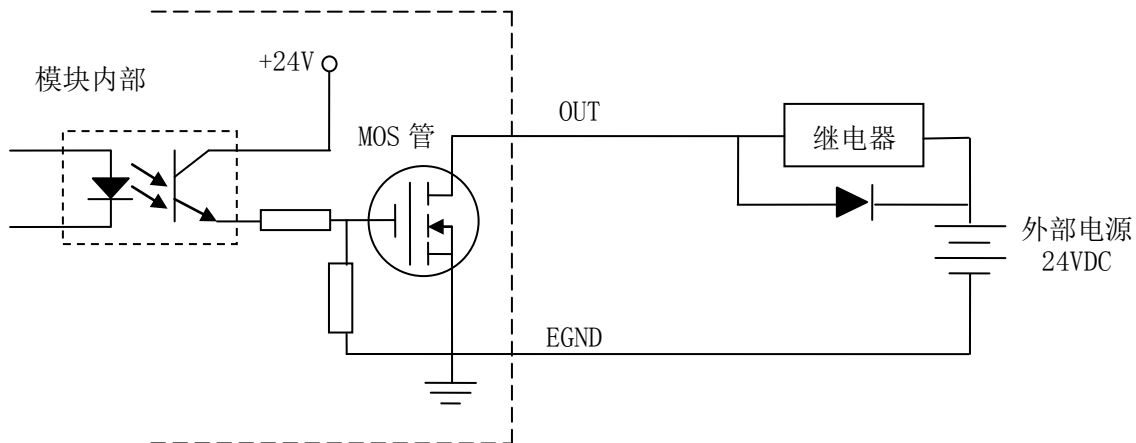
图 2.7 通用输出接线图
