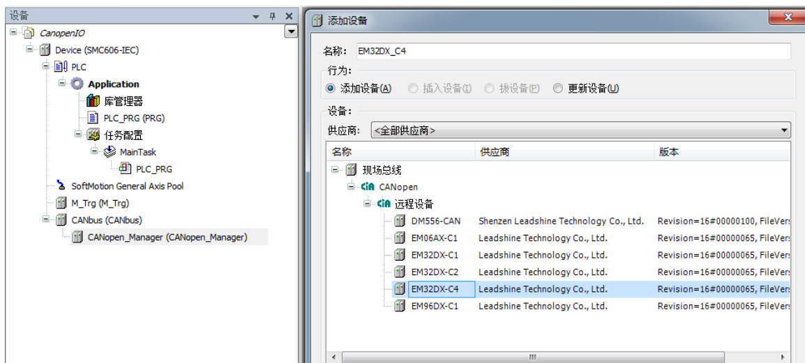
图 5.6 添加从站设备
