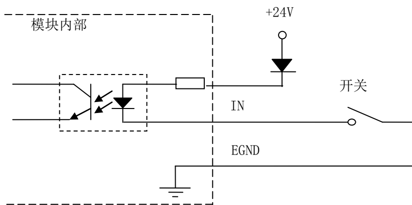
图 2.4 通用输入接线图
